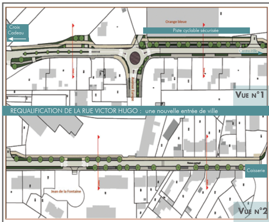
Projet d'aménagement de la rue V. Hugo avec création d'une piste cyclable sécurisée
